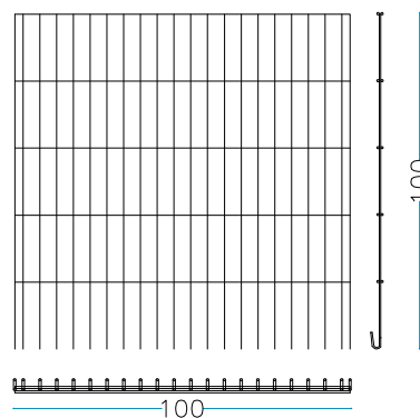
nr. 2 pz. Laterali corti 100 x H.100 cm
