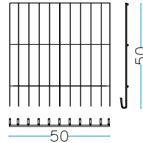
nr. 2 pz. Lateralì corti 100 x H.50 cm
