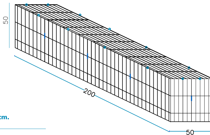
nr. 3 Tiranti interni L. 50 cm.
