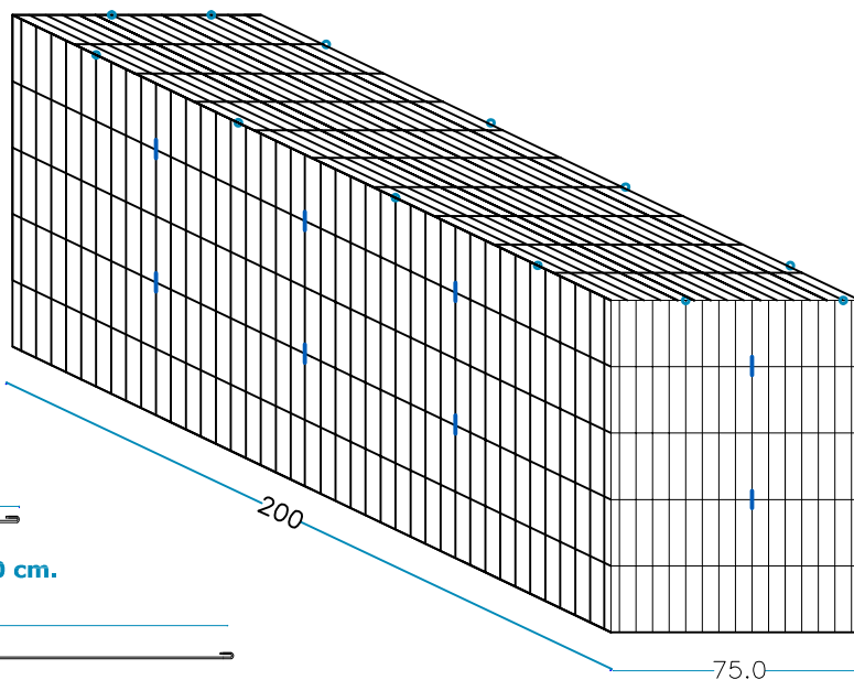
nr. 6 Tiranti interni L. 75 cm.
