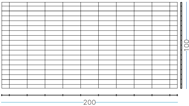
nr. 1 pz. Fondi 200 x 100 cm
