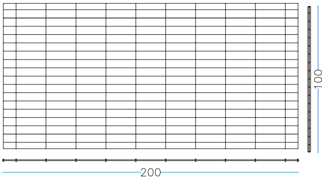
nr. 1 pz. Fondi 200 x 100 cm
