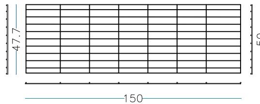
nr. 1 pz. Coperchi 150 x 50 cm
