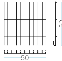
nr. 2 pz. Laterali corti 100 x H.50 cm
