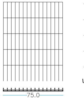
nr. 2 pz. Laterali corti 75 x H.100 cm
