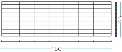
nr. 1 pz. Fondi 150 x 50 cm
