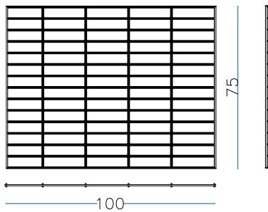
nr. 1 pz. Fondi 100 x 75 cm
