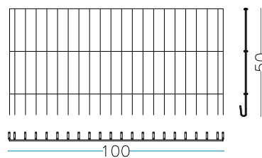
nr. 2 pz. Laterali corti 100 x H. 50 cm
