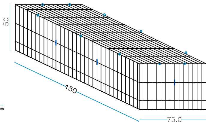
nr. 1 Tiranti interni L. 150 cm.
