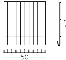
nr. 2 pz. Laterali corti 50 x H.50 cm
