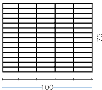
nr. 1 pz. Fondi 100 x 75 cm
