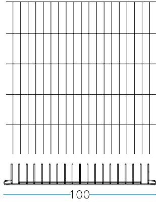
nr. 1 pz. Fondi 100 x 100 cm
