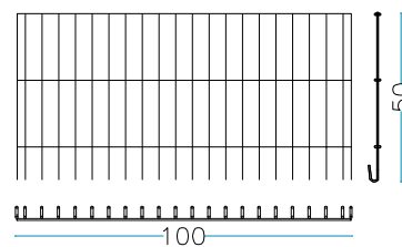
nr. 2 pz. Laterali corti 100 x H.50 cm
